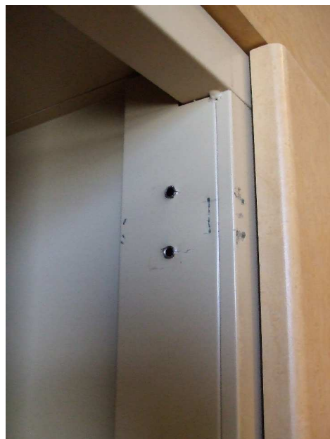
<原因>本体に取り付けたスライド蝶番 座金のビス穴が大きくなる
